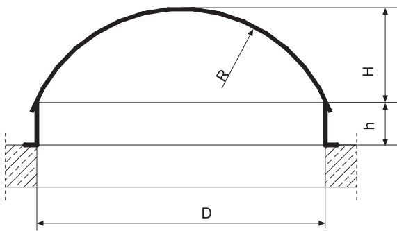
продольное сечение
